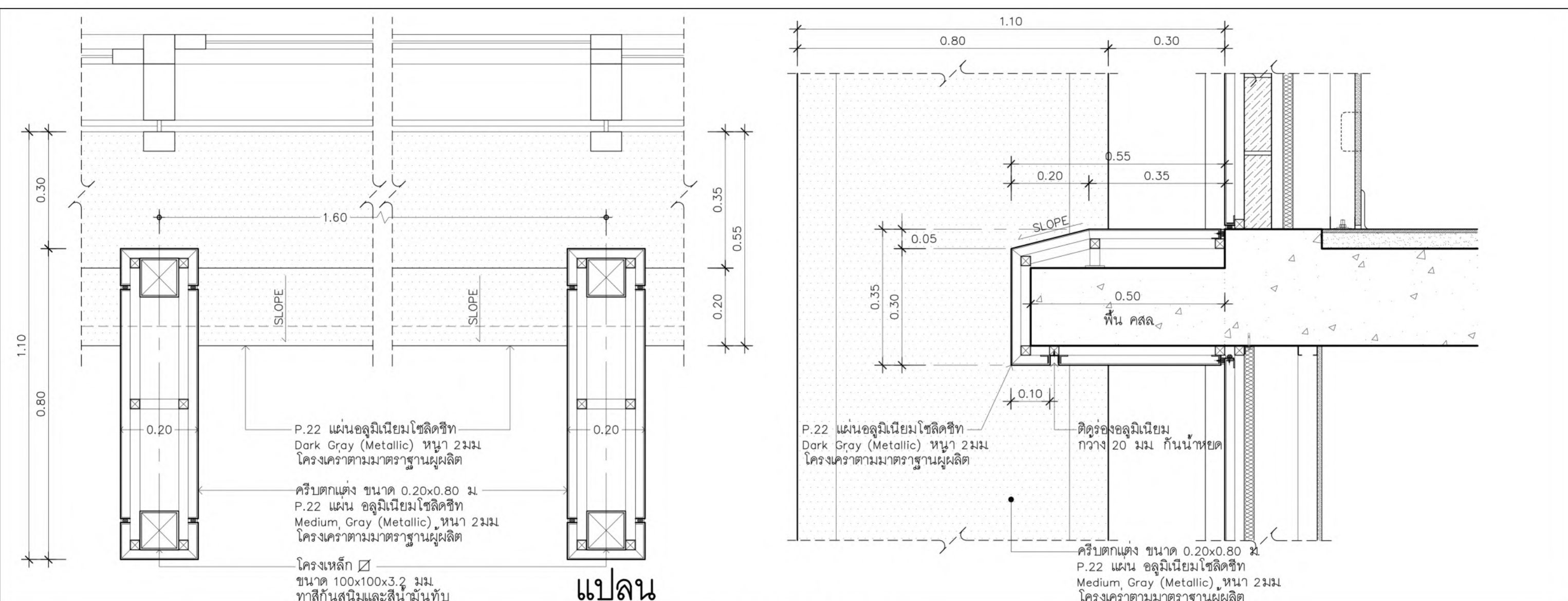
แบบขยาย FIN NO.8 มาตราส่วน 1:10
