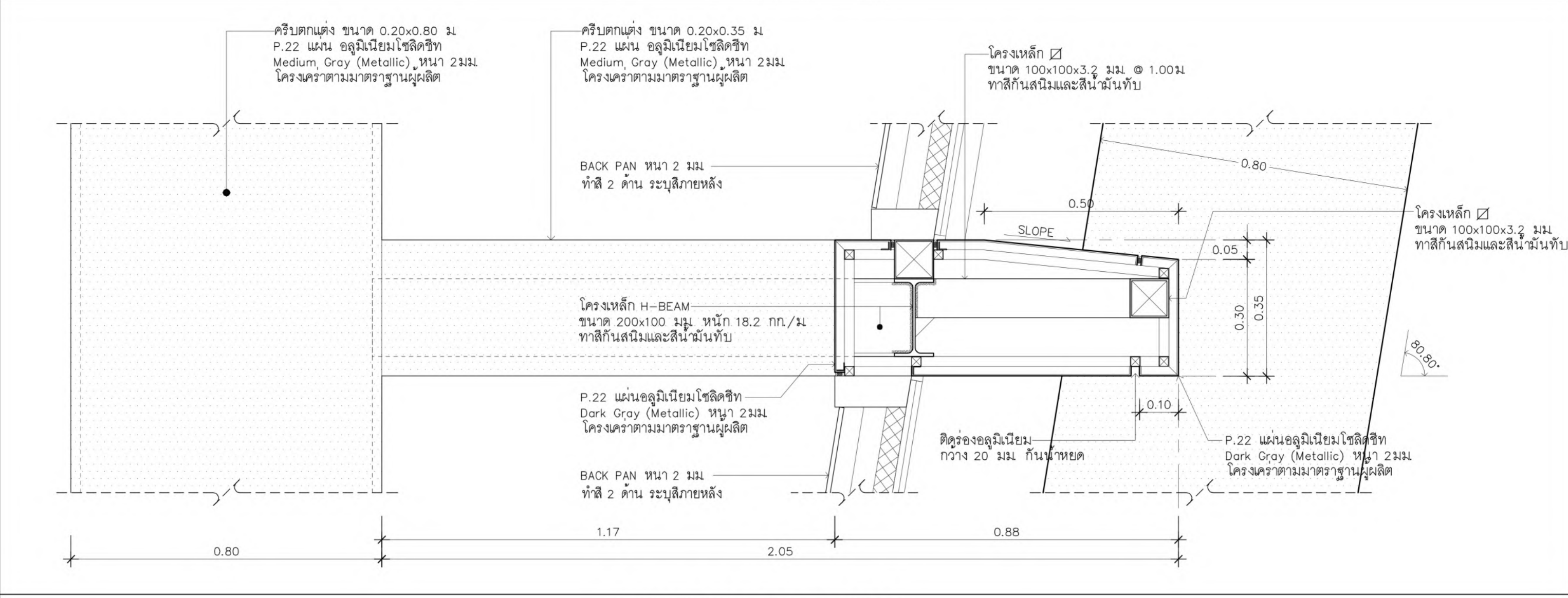
แบบขยาย FIN NO.1
