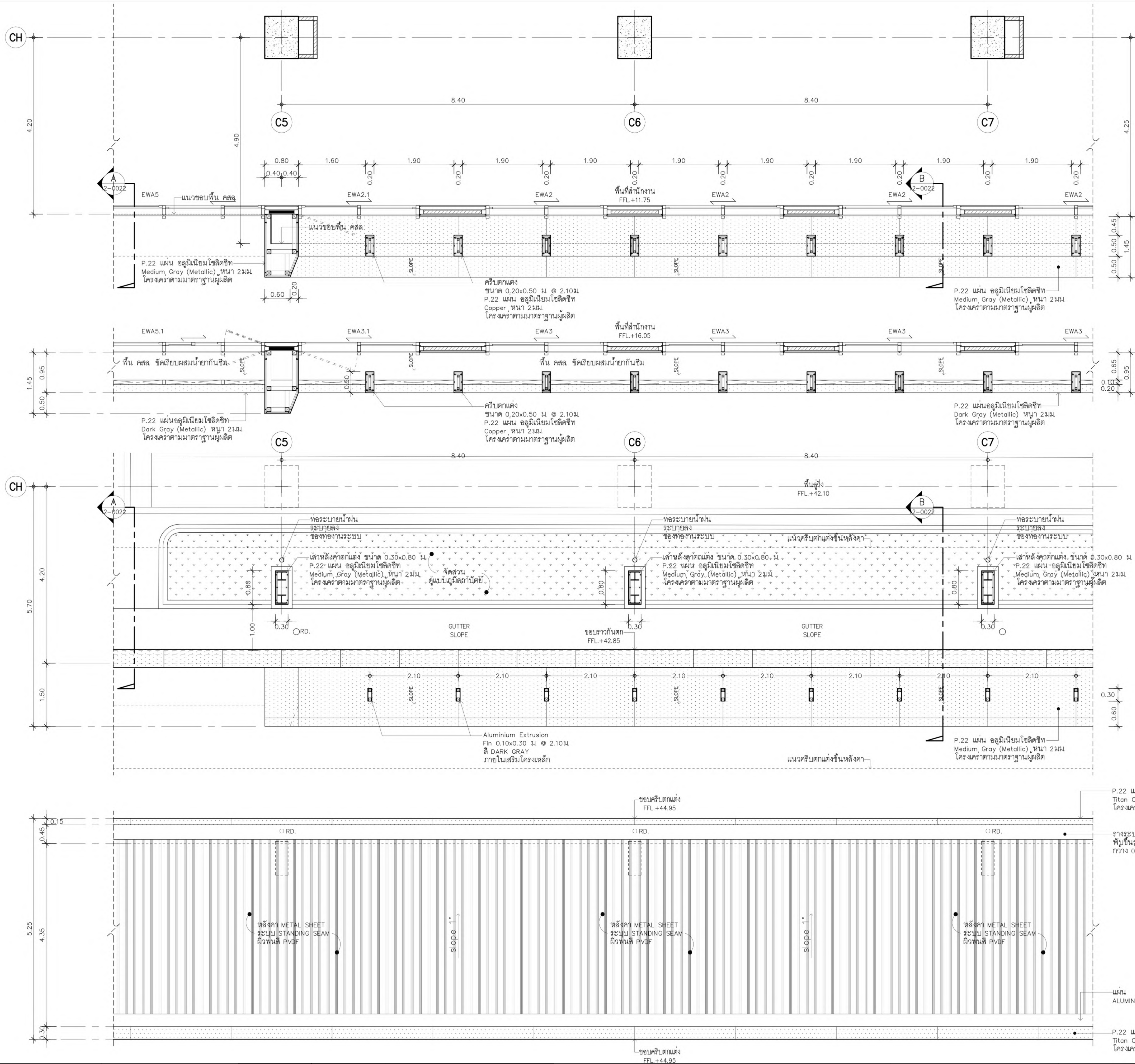
แปลนขยายรูปด้านคريبตกแต่ง 4 มาตราส่วน 1:50 ชั้นที่ 4
