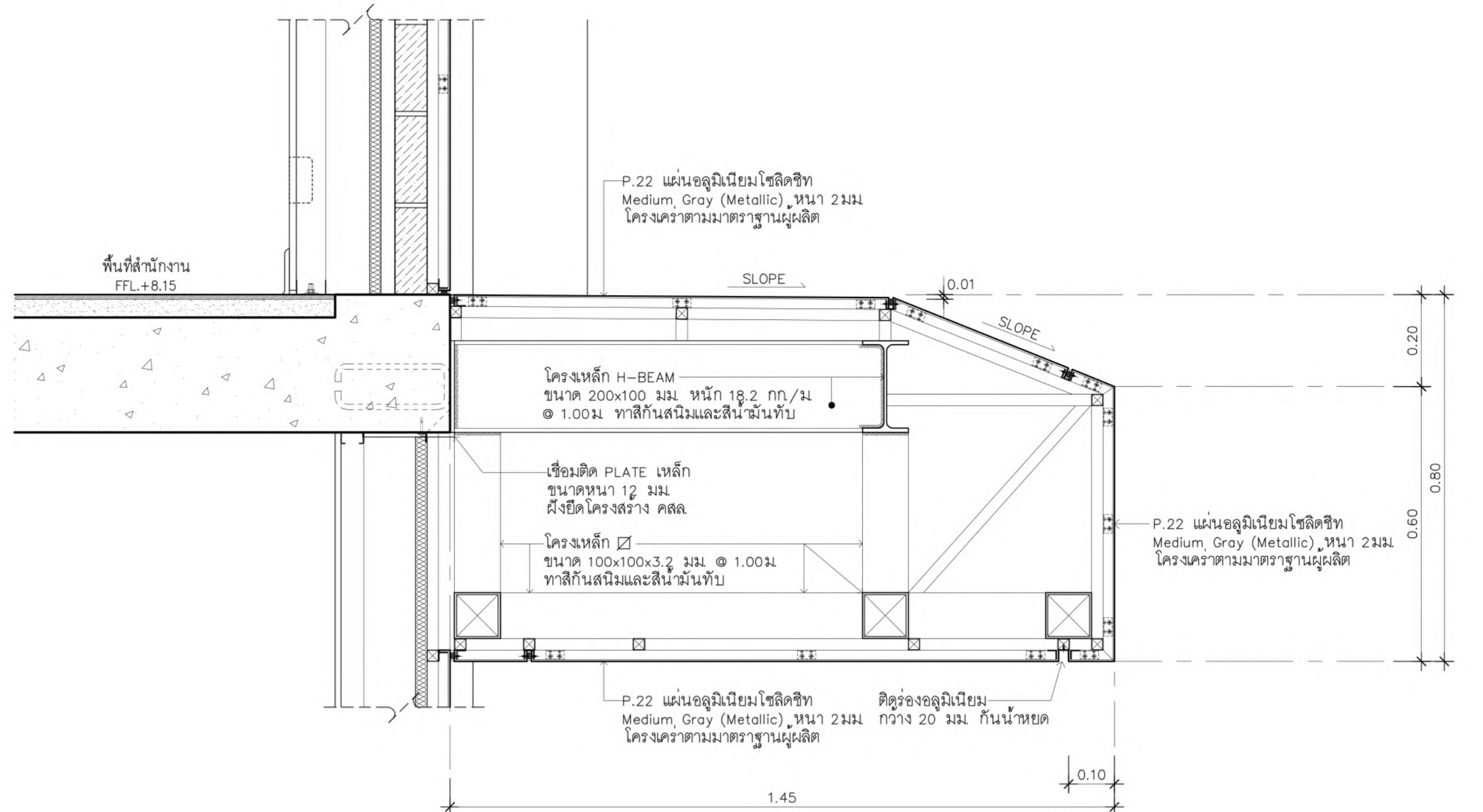
แบบขยาย FIN NO.4 มาตราส่วน 1:10
