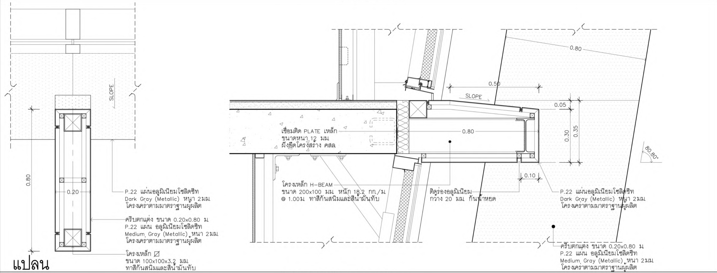
แบบขยาย FIN NO.9 มาตราส่วน 1:10
