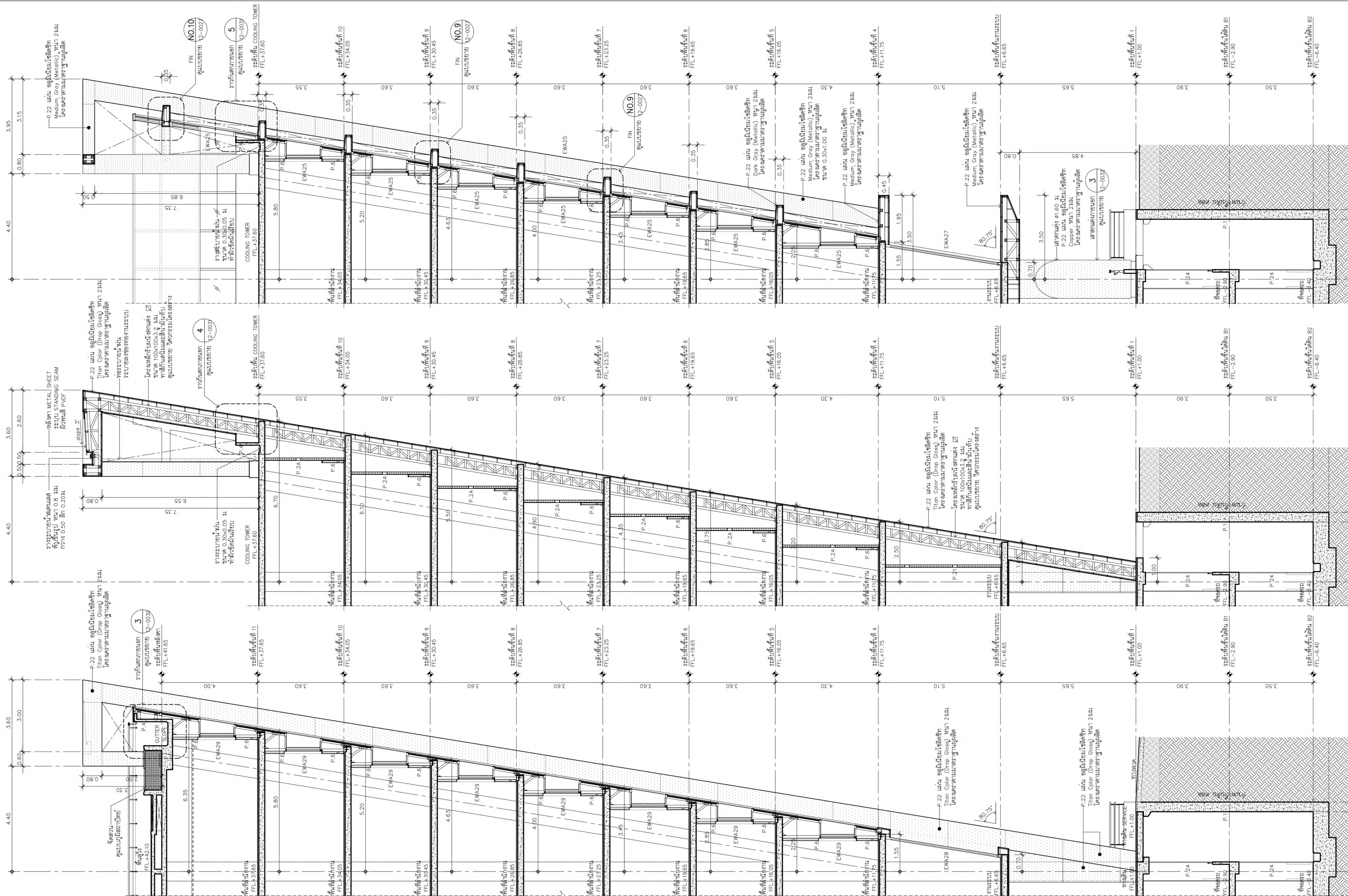
รูปตัดขยาย WS07 มาตราส่วน 1:75 C25
